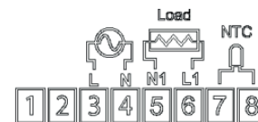
Схема подключения терморегулятора
