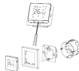
Схема подключения терморегулятора
